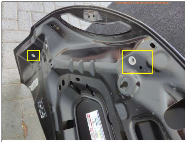
Bild 1: Altteil mit verbauten Gewindehülsen
